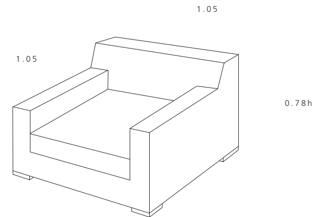
2006 - sillón ramsay original este fue el original, hecho para el estudio p.s.e. en la calle ramsay
